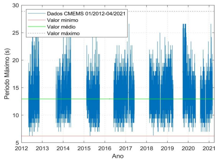
Figura 8.13 - Período máximo, boia ondógrafo de Ponta Delgada
