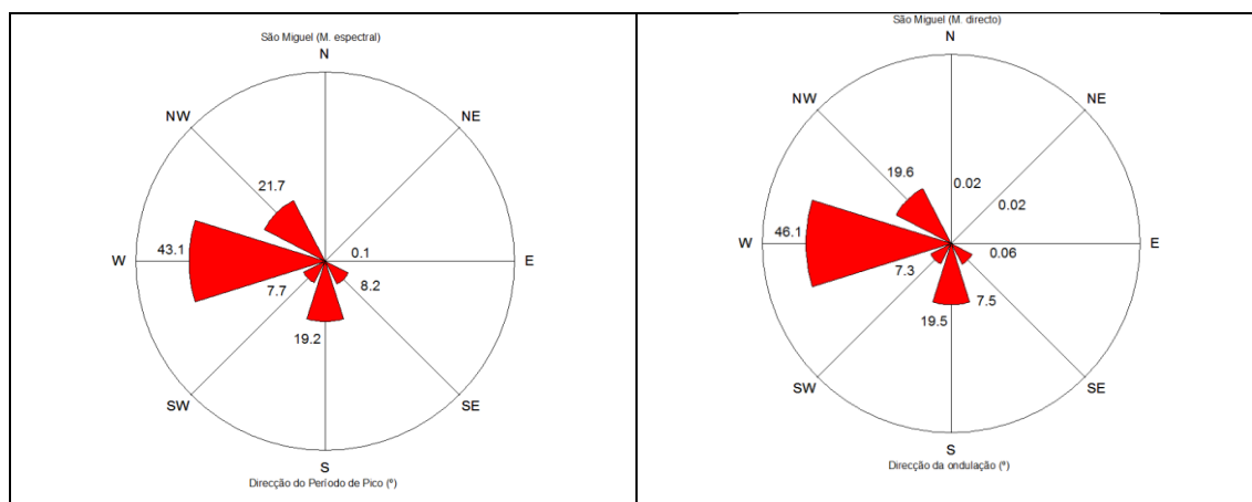
Figura 8.10 - Percentagem de ocorrências da direção da agitação marítima pelos métodos espectral e direto, em São Miguel
