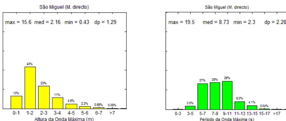
Figura 8.9 - Percentagem de ocorrências para a altura da onda máxima e o seu período associado, São Miguel
