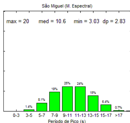
Figura 8.8 - Percentagem de ocorrências do período de pico pelo método espectral, em São Miguel
