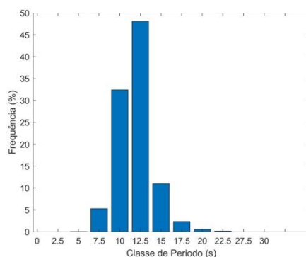
Figura 8.14 - Frequência do período máximo, boia ondógrafo de Ponta Delgada
