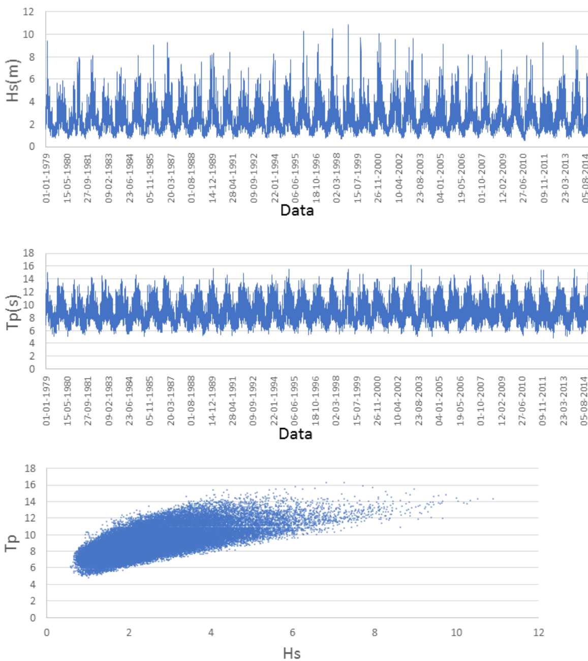
Figura 8.5 - Distribuição temporal de altura significativa [ H_s [m]], período de pico [ T_p [s]], e altura significativa em função do período de pico [ T_p ], ao longo dos 36 anos de estudo
