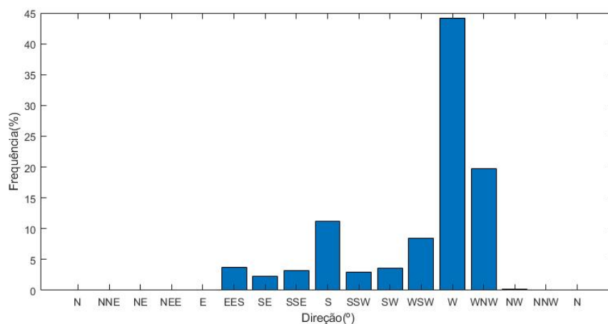
Figura 8.16 - Frequência da direção, boia ondógrafo de Ponta Delgada
