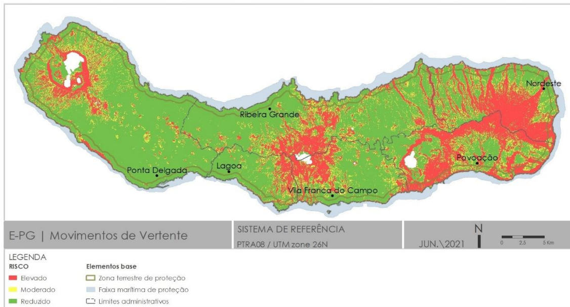
Figura 8.4 – Representação cartográfica das áreas de suscetibilidade à ocorrência de movimentos de vertente na ilha de São Miguel
