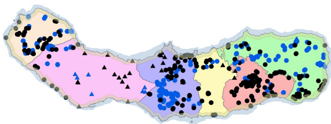
Figura 7.11 - Síntese da classificação do estado das massas de água subterrâneas na ilha de São Miguel
