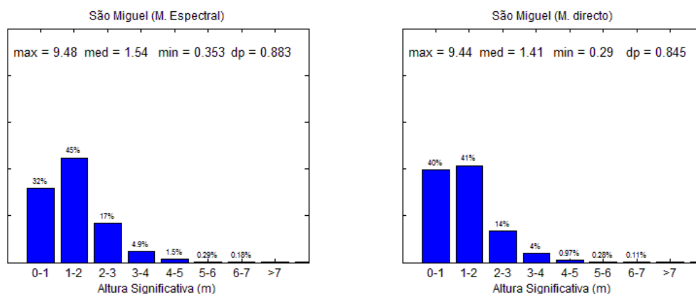
Figura 8.6 - Percentagem de ocorrências de altura significativa pelos métodos espectral e direto, em São Miguel
