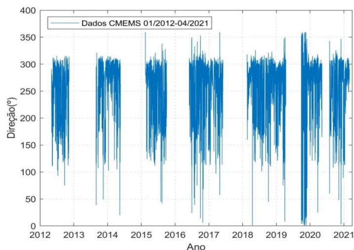
Figura 8.15 - Direção, boia ondógrafo de Ponta Delgada
