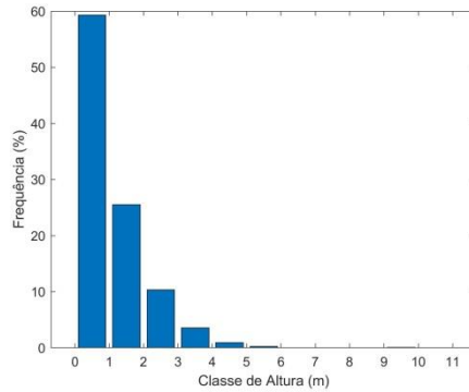
Figura 8.12 - Percentagem de ocorrências do terço das ondas mais altas, boia ondógrafo de Ponta Delgada
