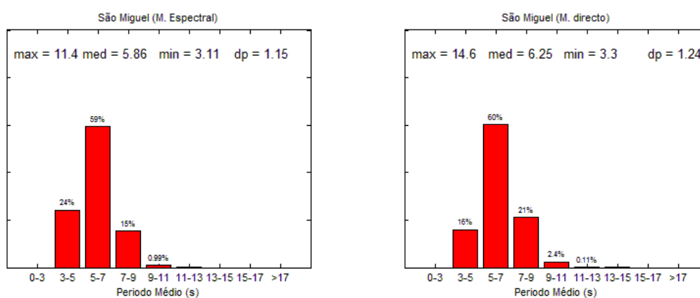
Figura 8.7 - Percentagem de ocorrências dos períodos médios pelos métodos espectral e direto, em São Miguel
