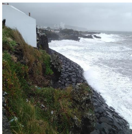
Setor com Enrocamento de suporte ao passeio marítimo e ciclovia de Lagoa Berma de proteção em enrocamento Atalhada
