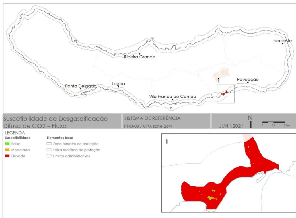
Figura 8.31 - Suscetibilidade de Desgaseificação Difusa de CO 2 – Concentração, na área de intervenção dos POOC_S Miguel
