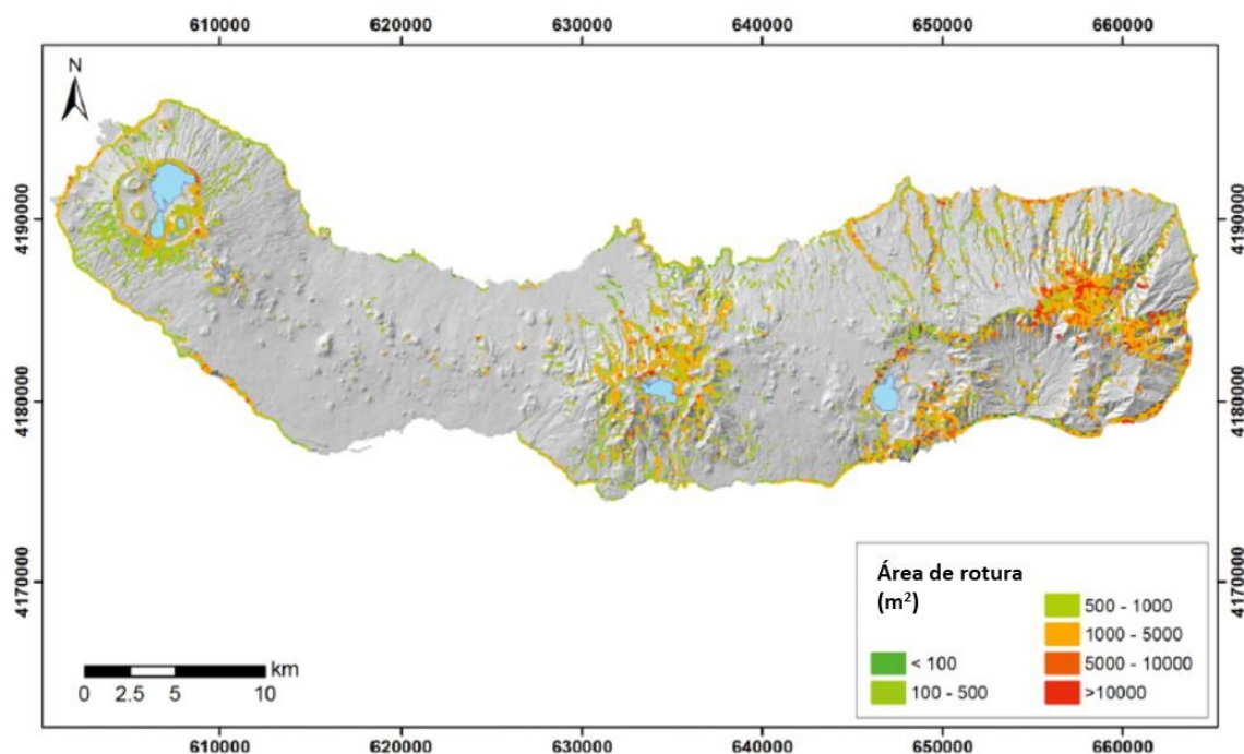
Figura 8.3 – Distribuição geográfica das áreas de rotura de movimentos de massa na ilha de São Miguel determinadas a partir de fotointerpretação
