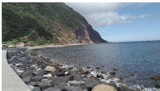
Obra longitudinal aderente com manto resistente em enrocamento – Faial da Terra, Povoação
